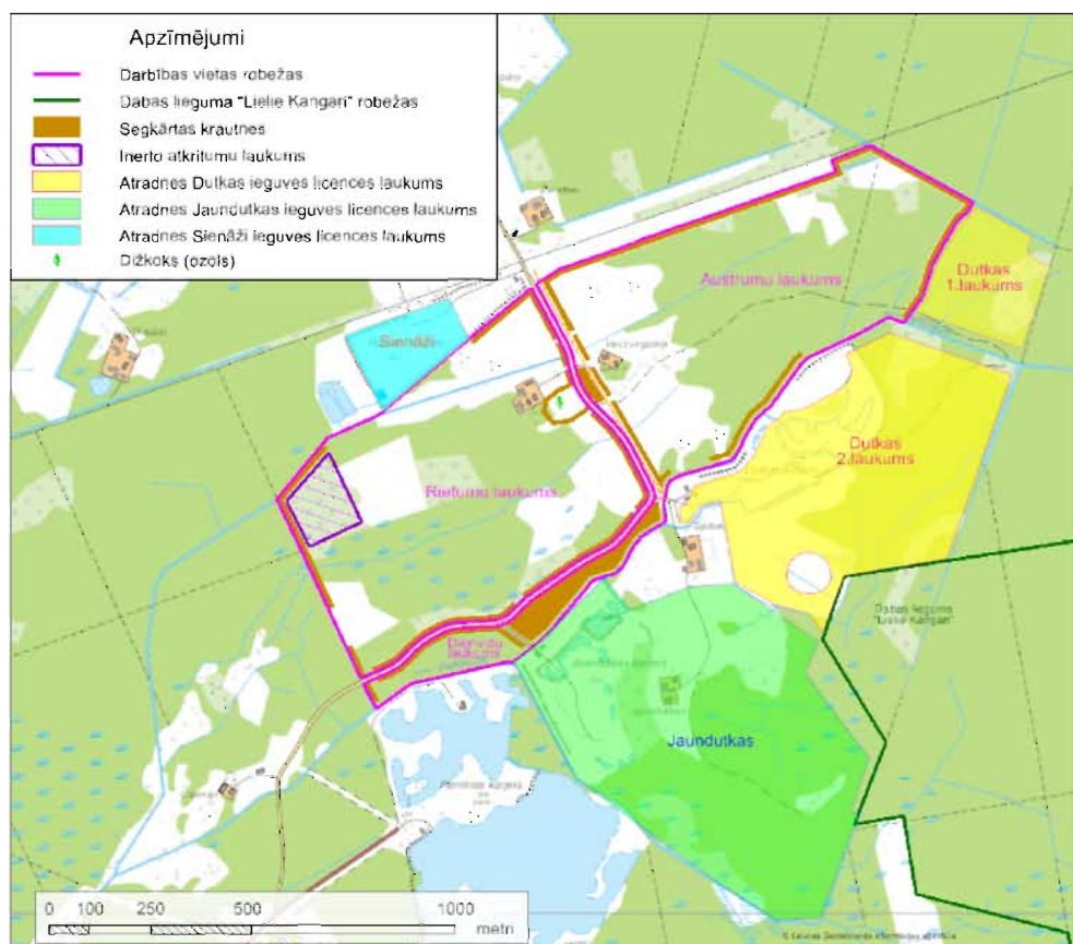
attēls. Inerto atkritumu pārstrādes un pagaidu uzglabāšanas laukuma izvietojums Darbības vietā
